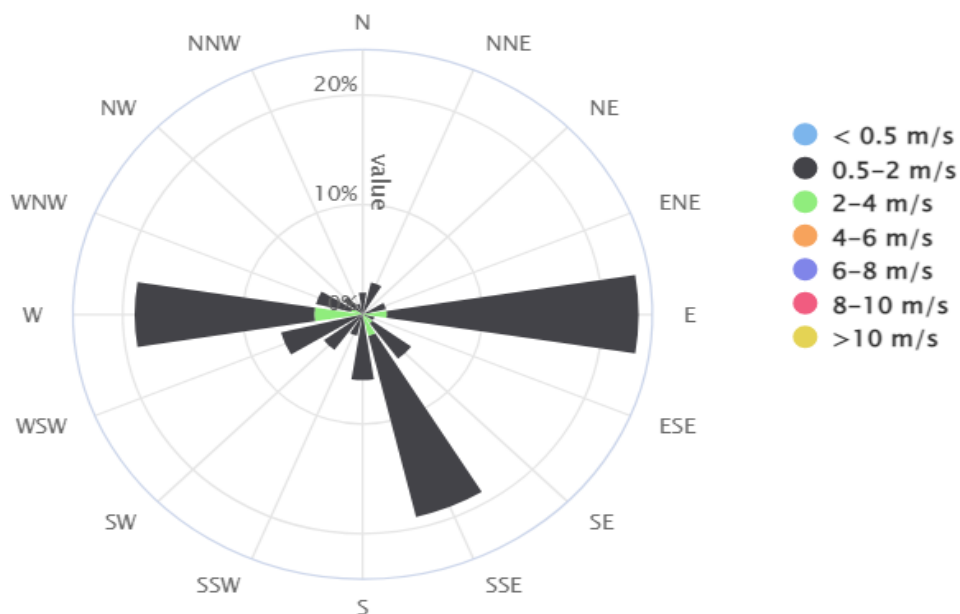
Rosa dei venti (classi di velocità)
