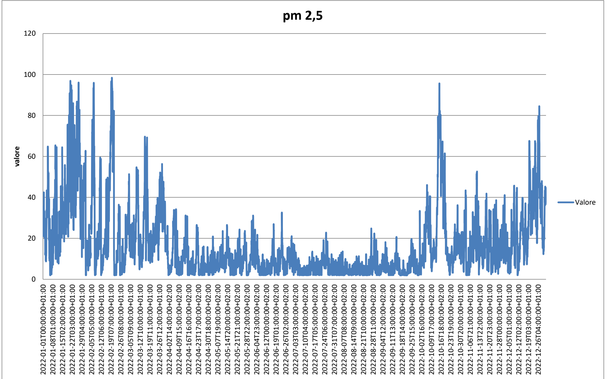
grafico PM2.5_tutto 2022
